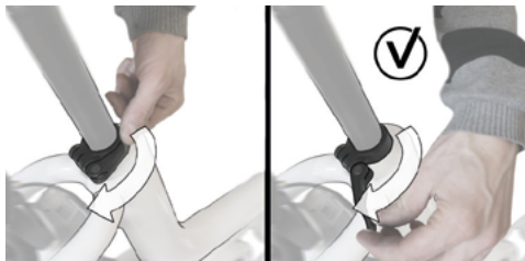
Abb. 6: Öffnen des Schnellspanners der Sattelstütze
